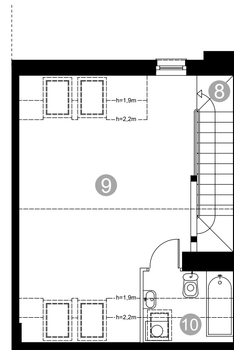
Poddasze
